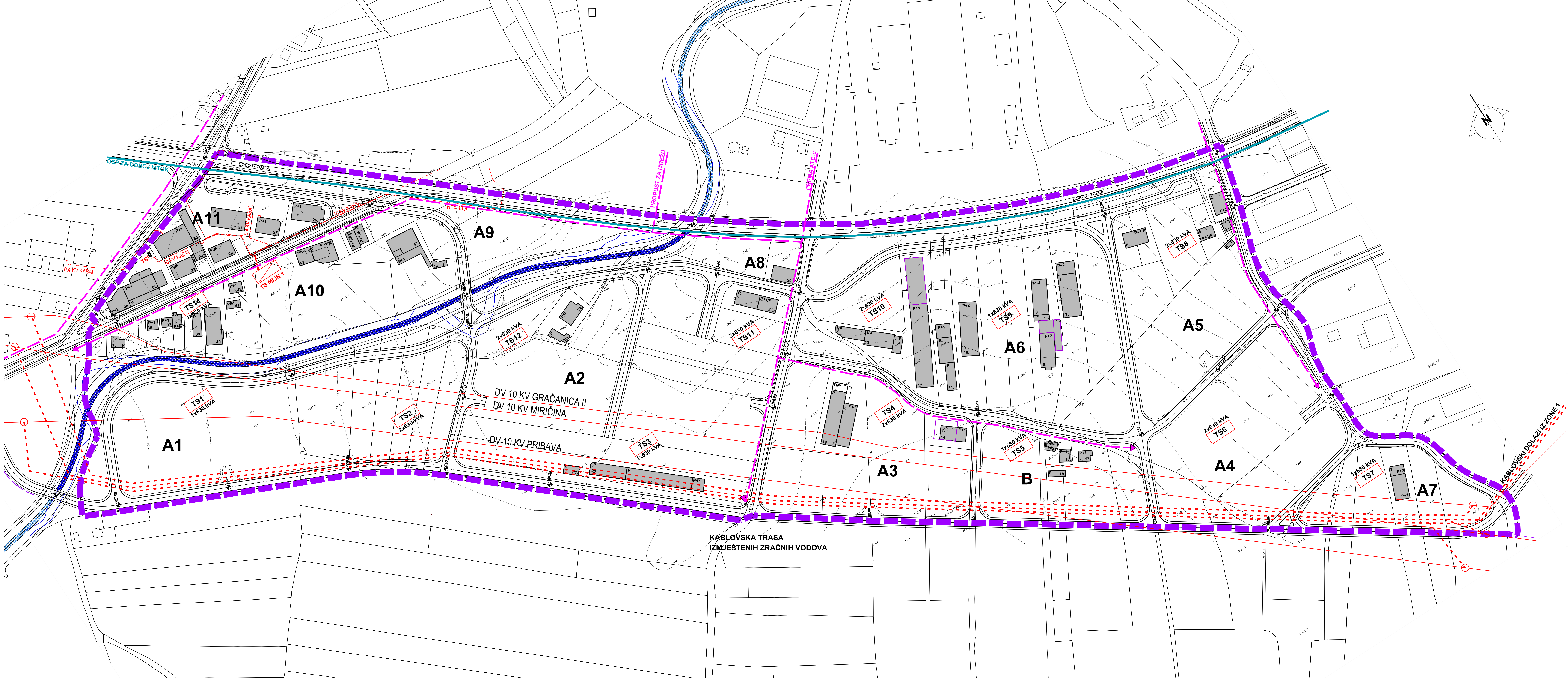
ŠEMA VEZE TS 10(20)/0,4 KV U RADNOJ ZONI II
